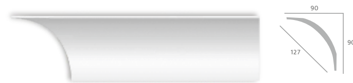
PCN-2100 240 x 9 x 9 cm
